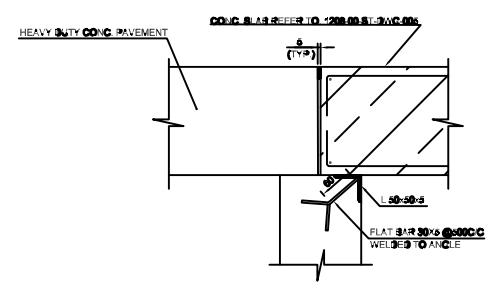
DET. "2" (C 1) SC 120
